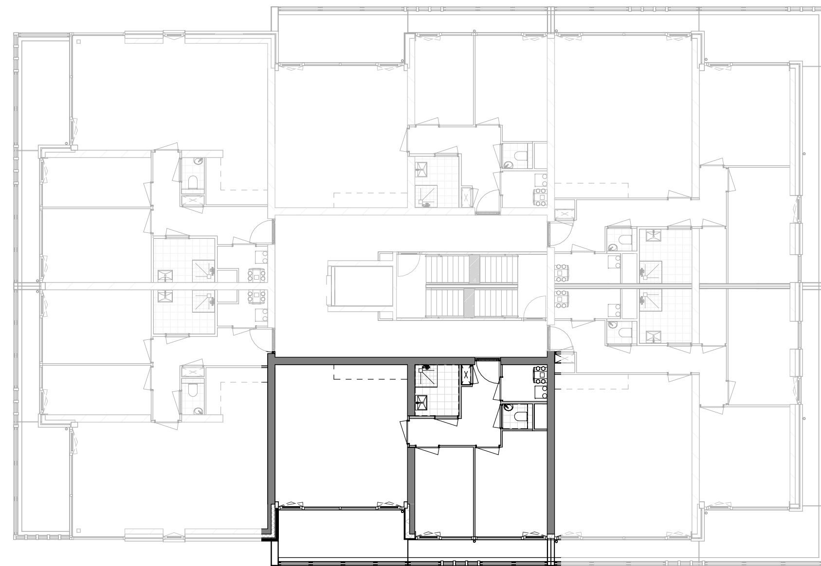
Tweede verdieping 0 1 : 150
