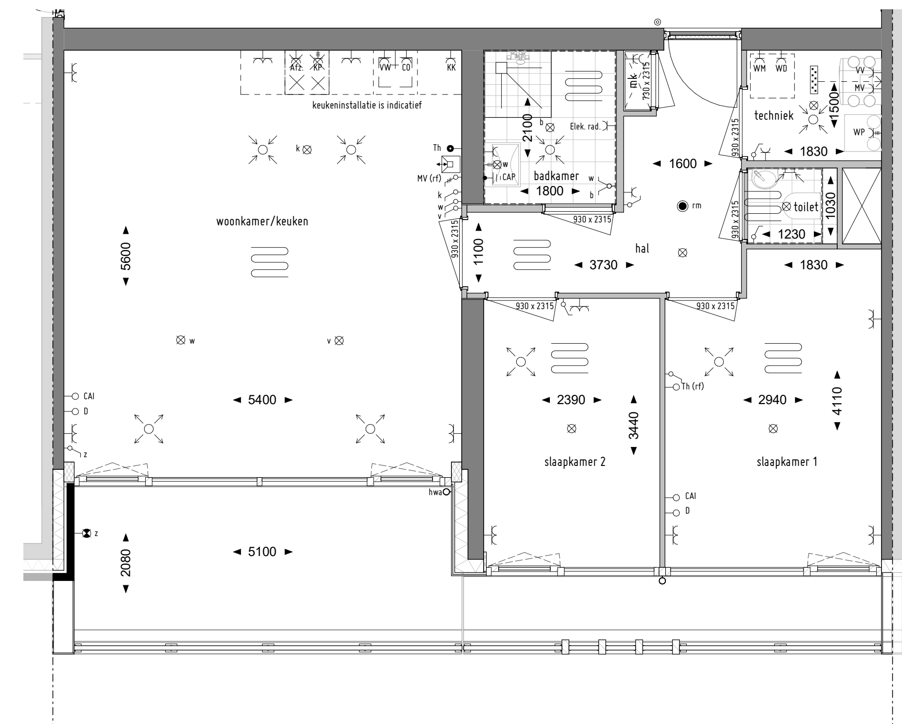
Tweede verdieping 0 1 : 50
